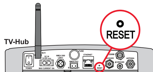
Figure 37: TV-Hub Reset Button
